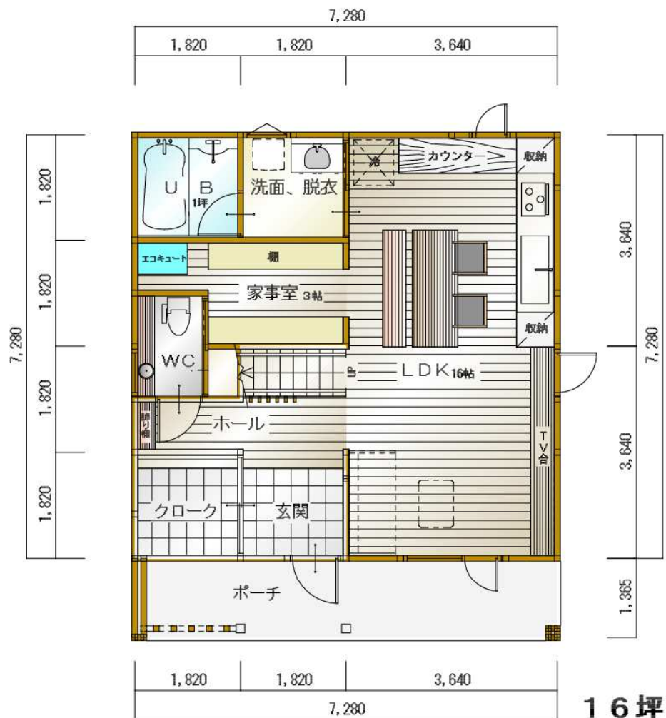
1階 平面図
