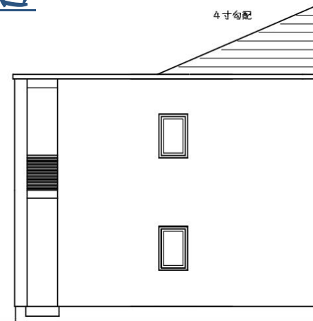
東面立面図
