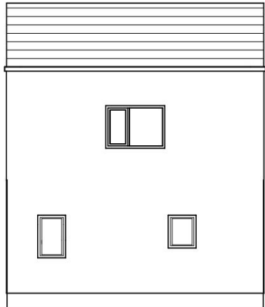
北面立面図
