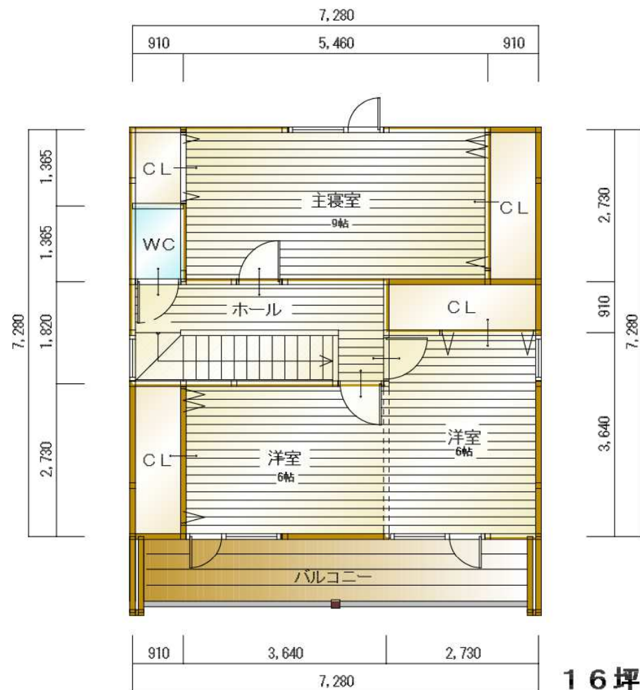
2階 平面図
